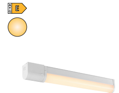
Malaika 49 2310201001 White | Aluminium LED Module 6W | 540lm | 3000K H: 7 cm | W: 5,5 cm | L: 49,4 cm
